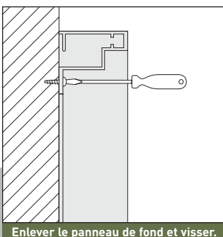
Enlever le panneau de fond et visser.
