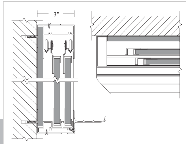
Mécanisme vu de profil
