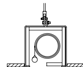
Fixation encastrée
