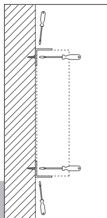
Installation des équerres continues
