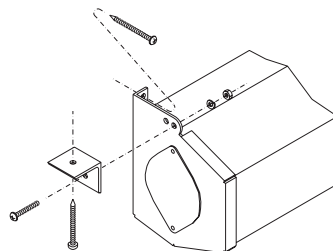
Fixation plafond suspendu
