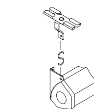
Fixation plafond suspendu
